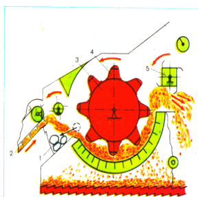
Рис. 37 Молотильное устройство комбайна «Дон-1500»: 1 — камнеуловитель; 2 — плавающая транспортер; 3 — молотильный барабан; 4 — подбарабан; 5 — отбойный битер
