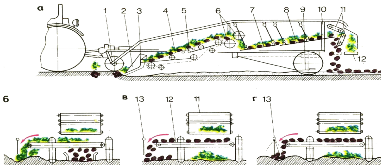
Рис. 124. Технологическая схема работы картофелекопателя-валкоукладчика УКВ-2: а — схема работы, б — укладка клубней «вслед», в, г — вынос клубней на сторону; 1 — опорное колесо, 2 — активная боковина, 3 — лемех, 4 — основной элеватор, 5 — встряхиватель, 6 — комкодавитель, 7 — первое решето грохота, 8 — второе решето грохота, 9 — ложеобразователь, 10 — ботвоотделяющие трости, 11 — поперечный конвейер, 12 — ботвоудалитель, 13 — щиток
