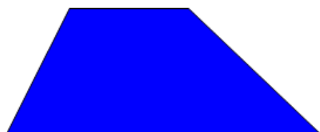
Трапедия
