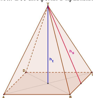
Правильная пирамида
