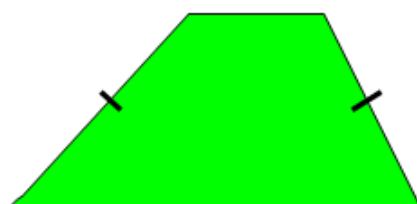
Произвольная трапедия
