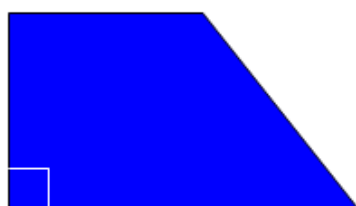
Прямоугольная трапедия
