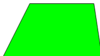
Произвольная трапедия
