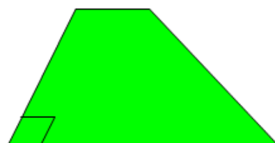
Произвольная трапедия
